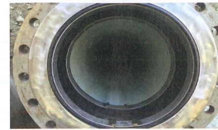
Ergebnis der erfolgreichen Sanierung: ein neues Rohr, dessen Qualität den hohen Anforderungen einer Herstellung im Werk entspricht.
