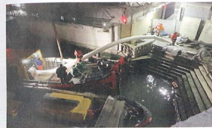
Der BlueLiner musste aus der Inversionstrommel heraus in einem weiten Bogen zur Leitung geführt werden.
